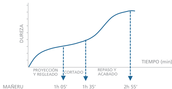
Evolución media de fraguado
