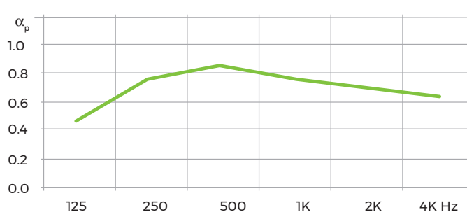
■ Plenum de 200
